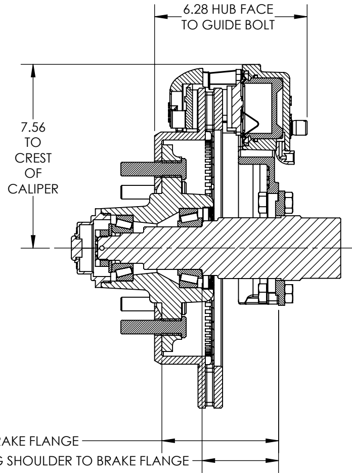
SECTION A-A
