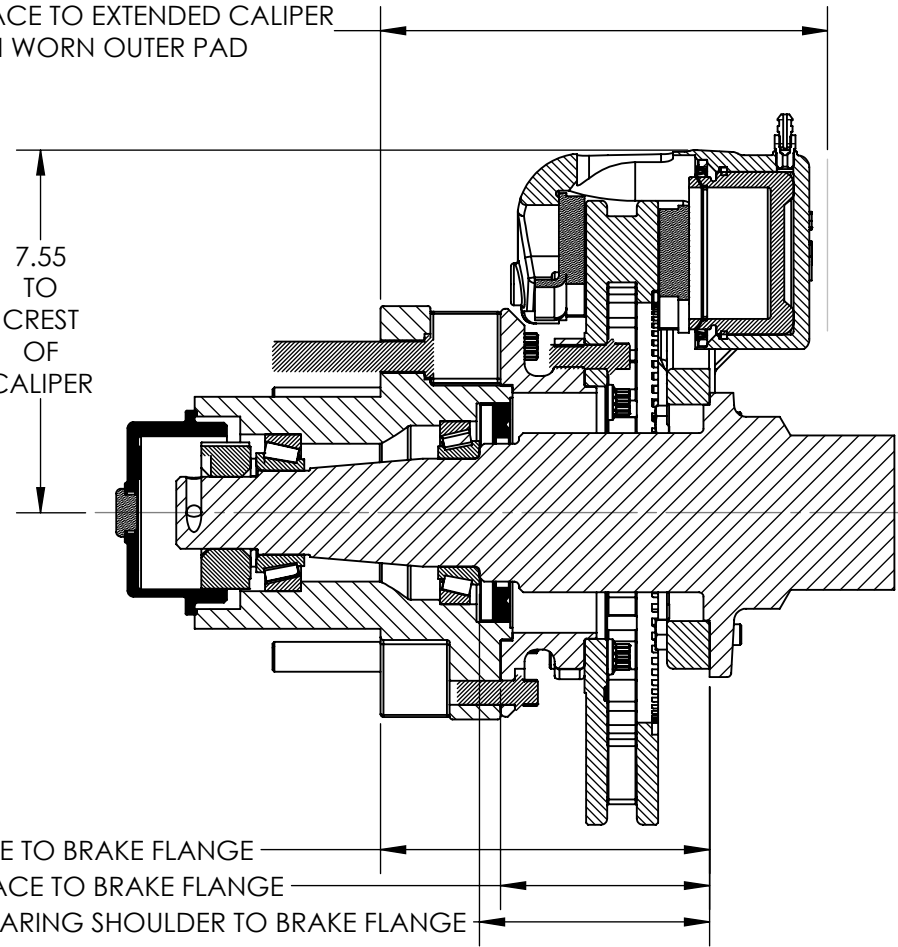
SECTION A-A
