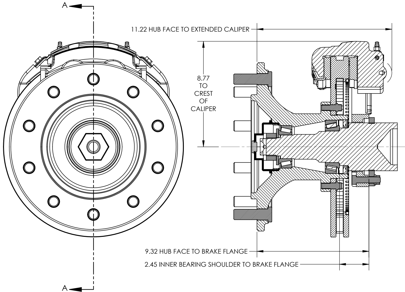
SECTION A-A
