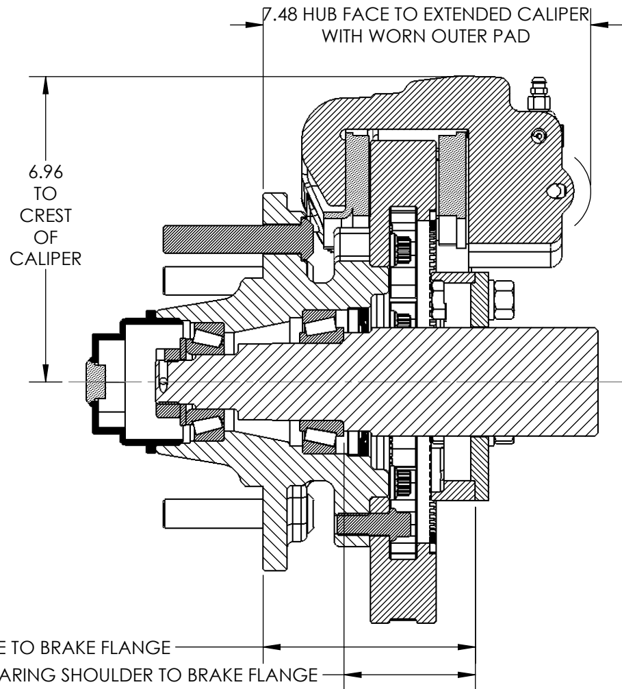
SECTION A-A
