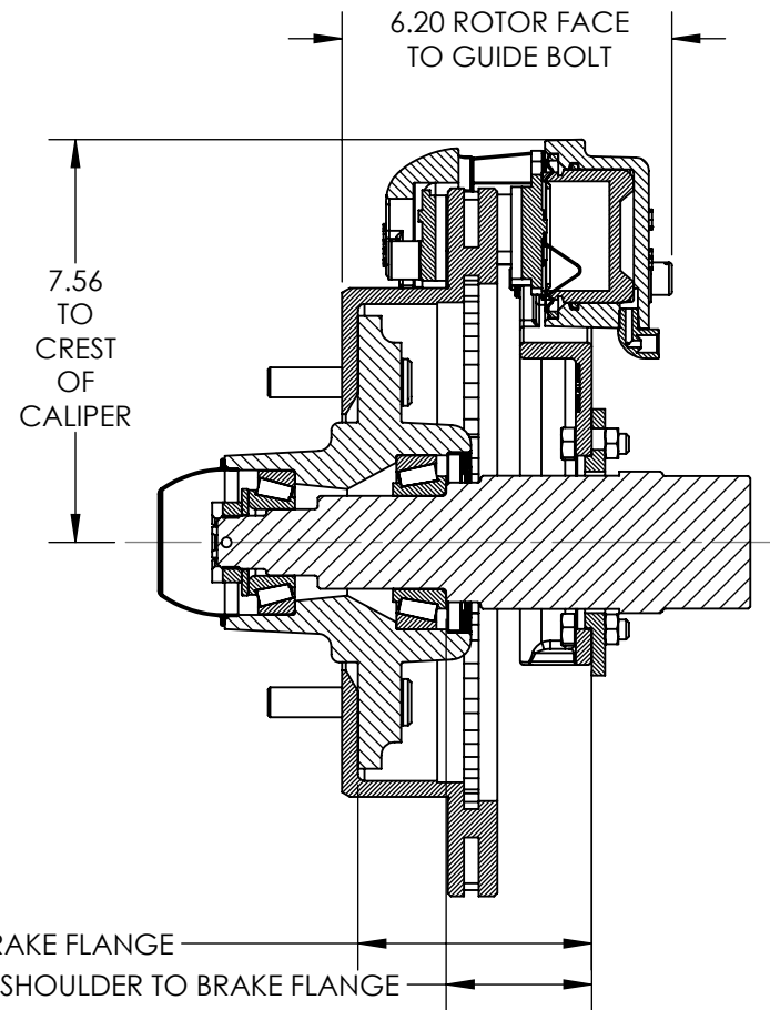
SECTION A-A
