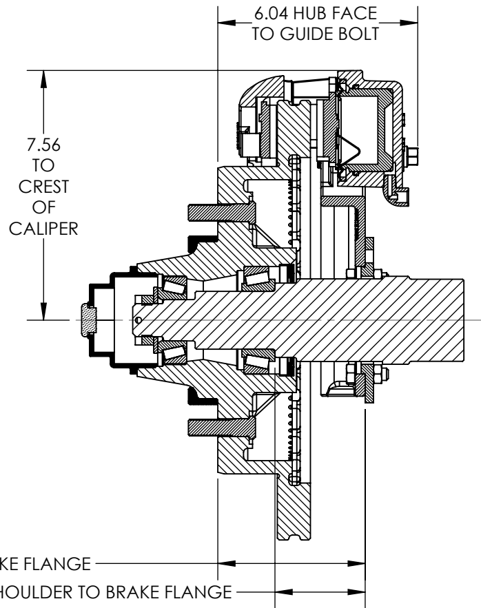
SECTION A-A
